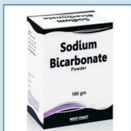
SODIUM BICARBONATE
